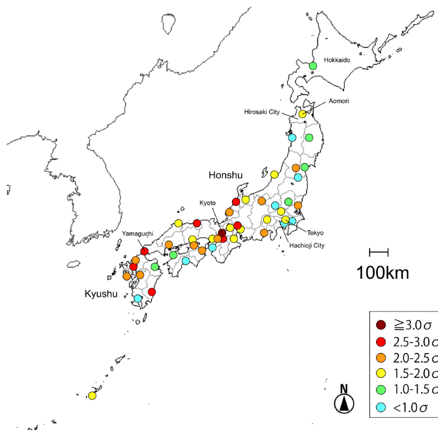
図 2：現代の雷データ（1989～2014 年）による 27 日周期の強度マップ。 \sigma は統計的有意性を示す値で、数値が高いほど有意性が強い（偶然性が低い）ことを示す。例えば、 1.5\sigma が 86% の有意性（すなわち、偶然に起こる確率が 14%）、 2.0\sigma が 95% の有意性（偶然に起こる確率が 5%）を示している。出典：Miyahara H., et al. Ann. Geophys., 36, 633-640, 2018
