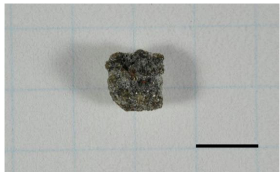
図 1：分析した隕石。図中の黒線は 5 mm。国立科学博物館所蔵
